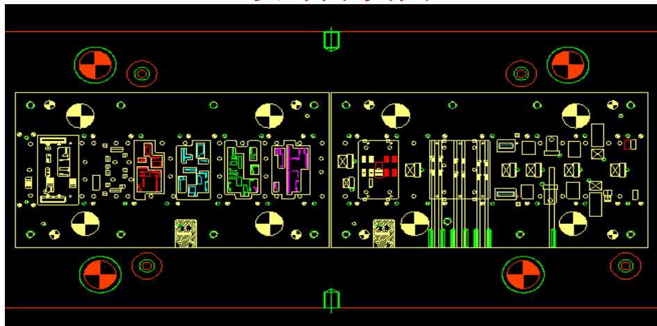
设计开发图
