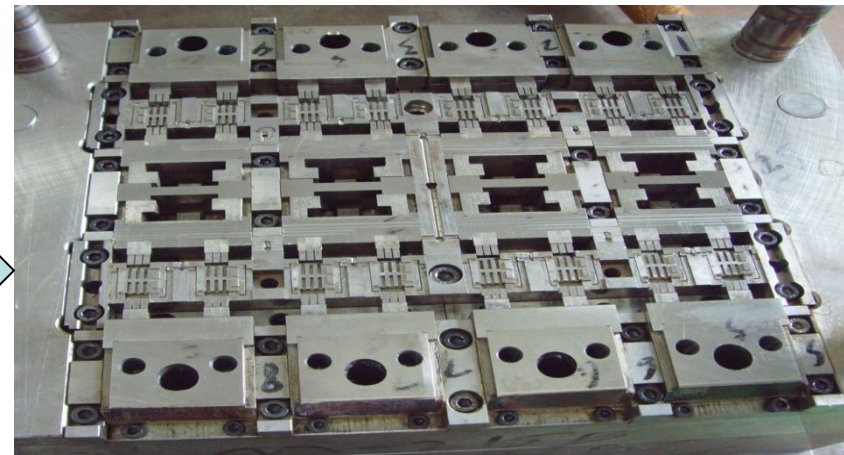
设计实现图
