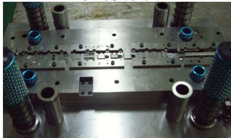
设计实现图
