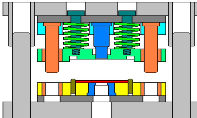
设计实现图
