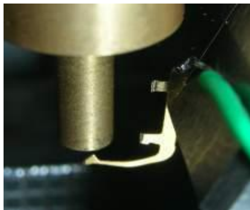
插拔力测试
