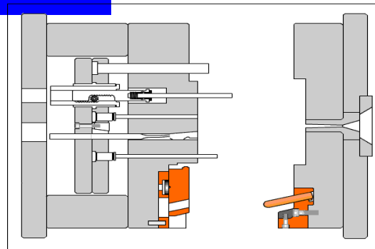
设计实现图
